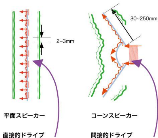
従来型コーンスピーカーとの比較
